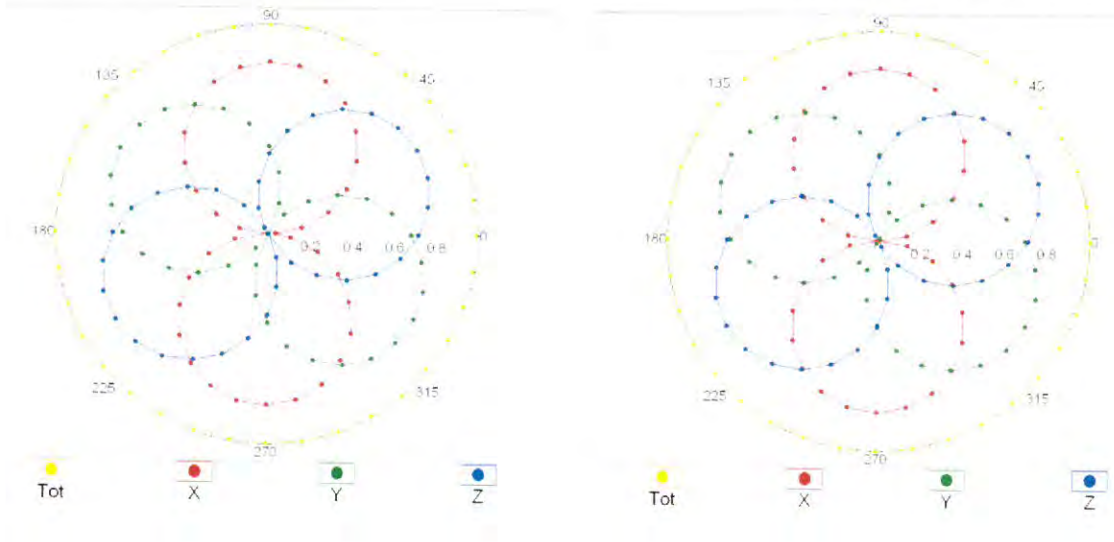
f=1800 MHz,R22
