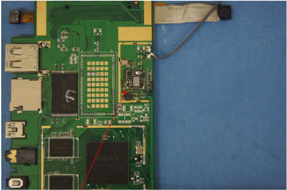
Wifi module
