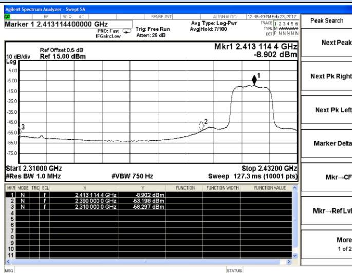
802.11n(HT20)-Low channel(Average)
