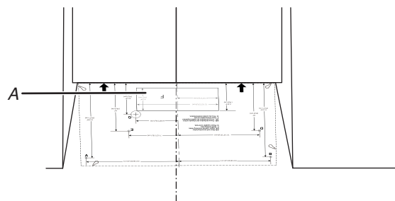
A. Área de recorte de la ventilación a través de la pared
