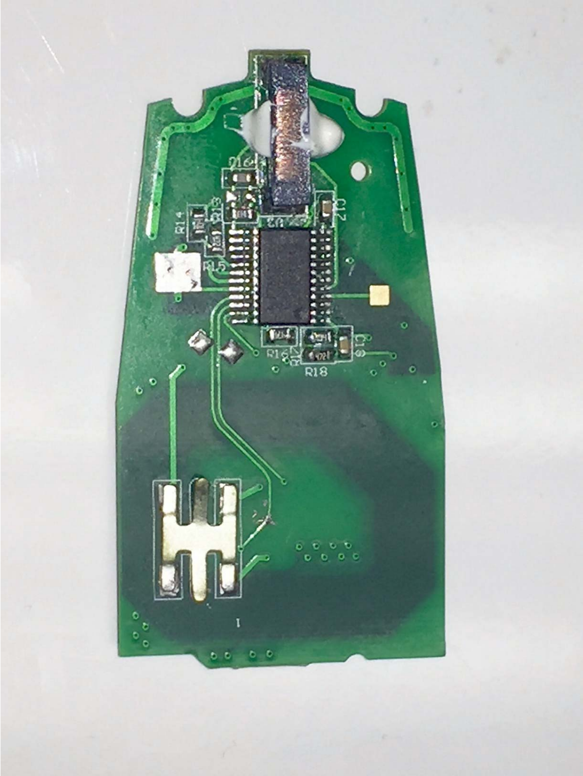
PCB Bottom
