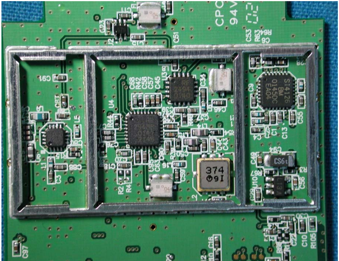
(5) EUT Photo
