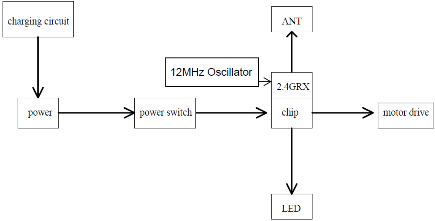
66804RXV12-block diagram
