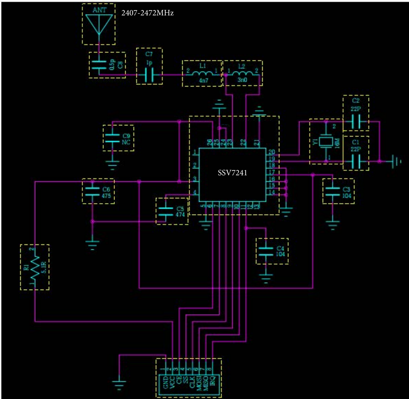
RF Module WT24DK2015
