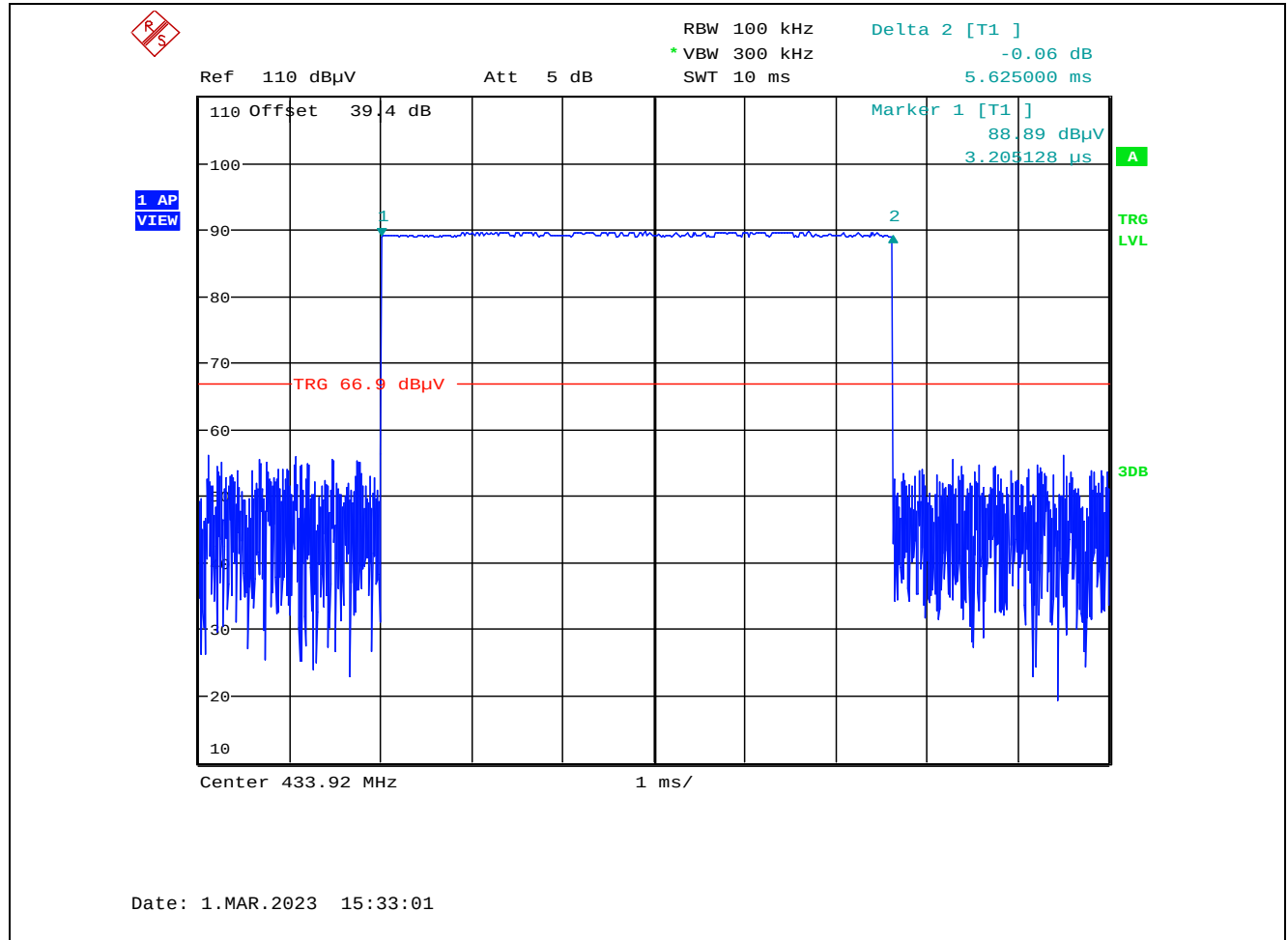
Plot 5.2.3.3.3. Duty Cycle (Pulse)
