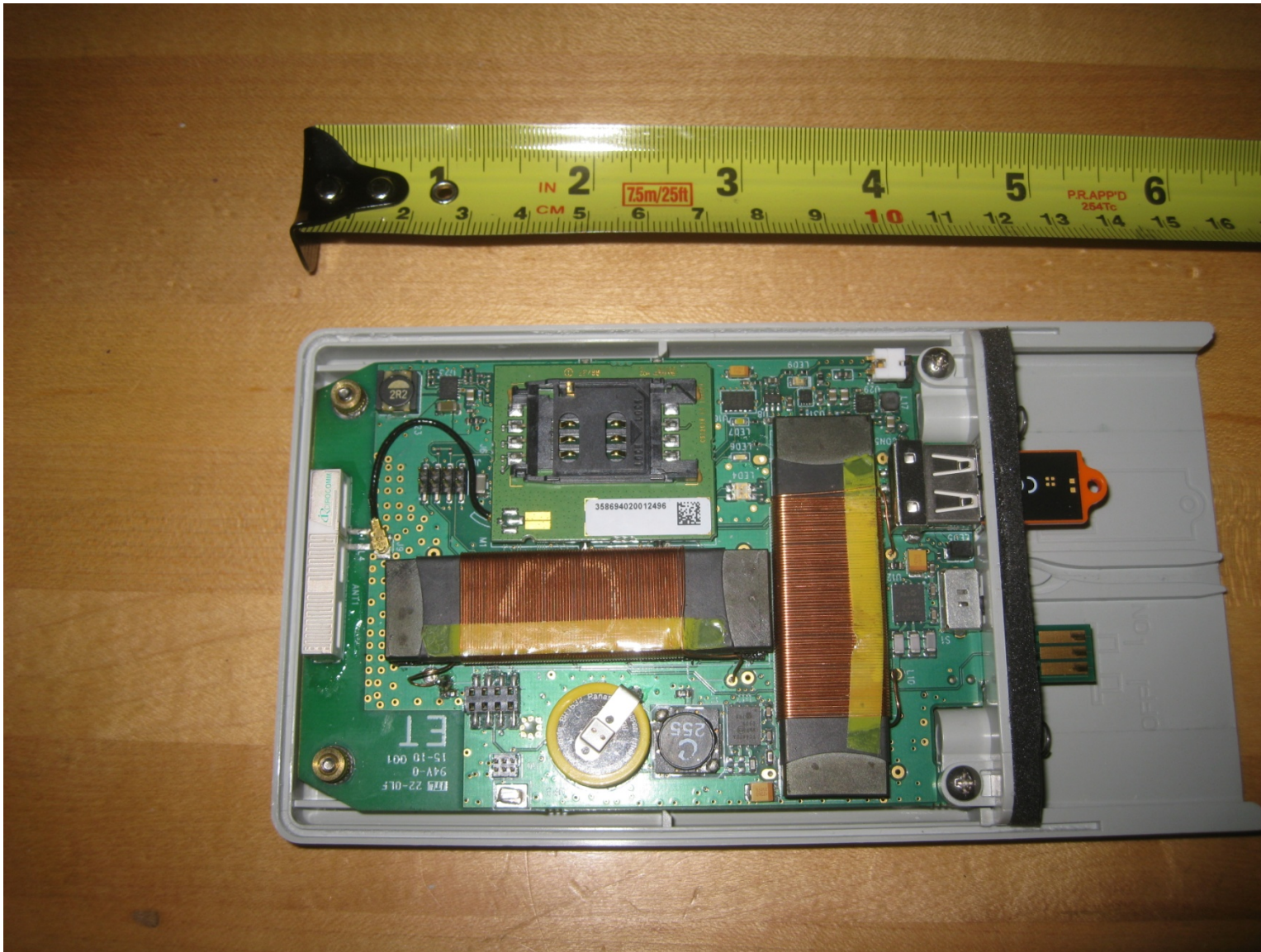
Top Side
