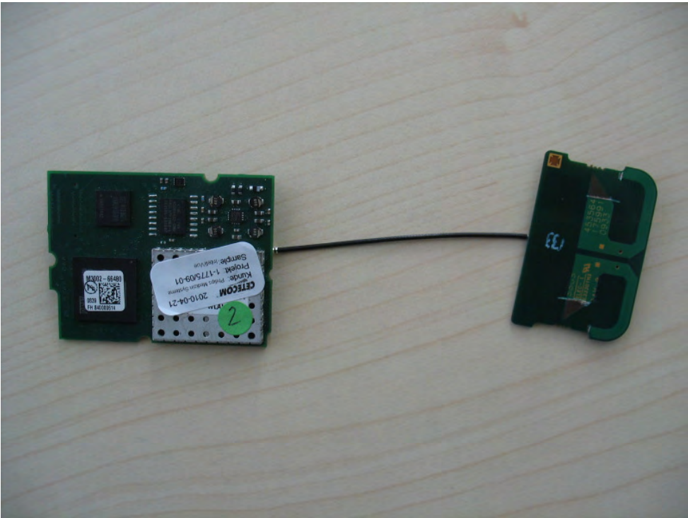
Photo 3: (WLAN Module / Antenna):
