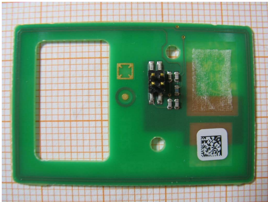
Photo 4: EUT
