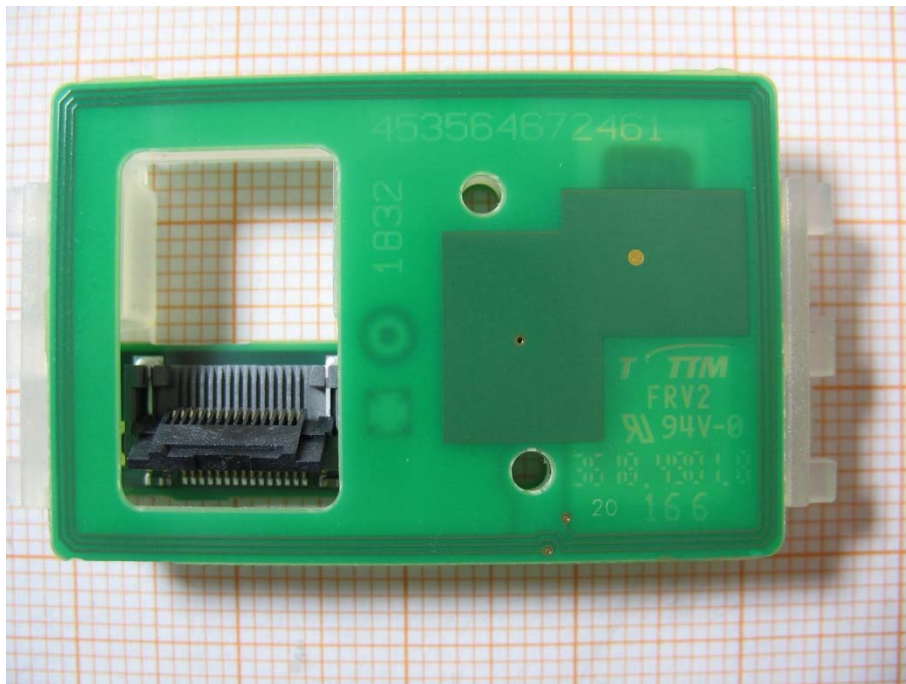
Photo 2:EUT
