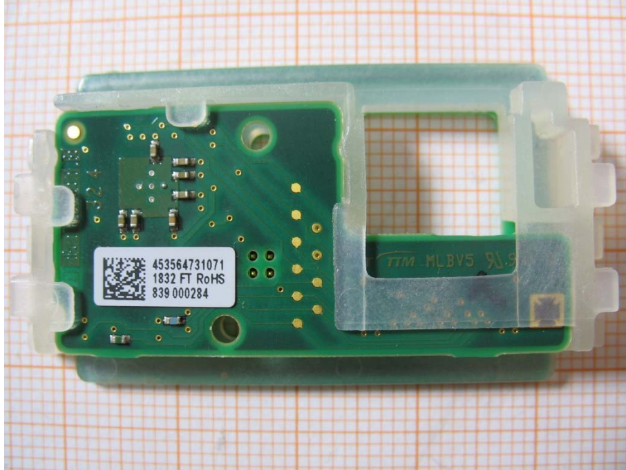
Photo 3: EUT
