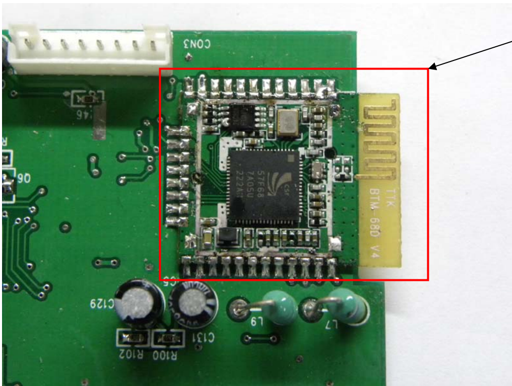
RF Module 1
