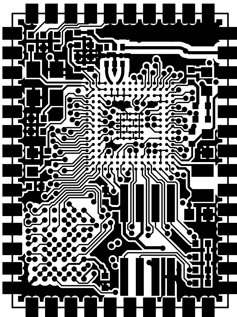
Top Layer
