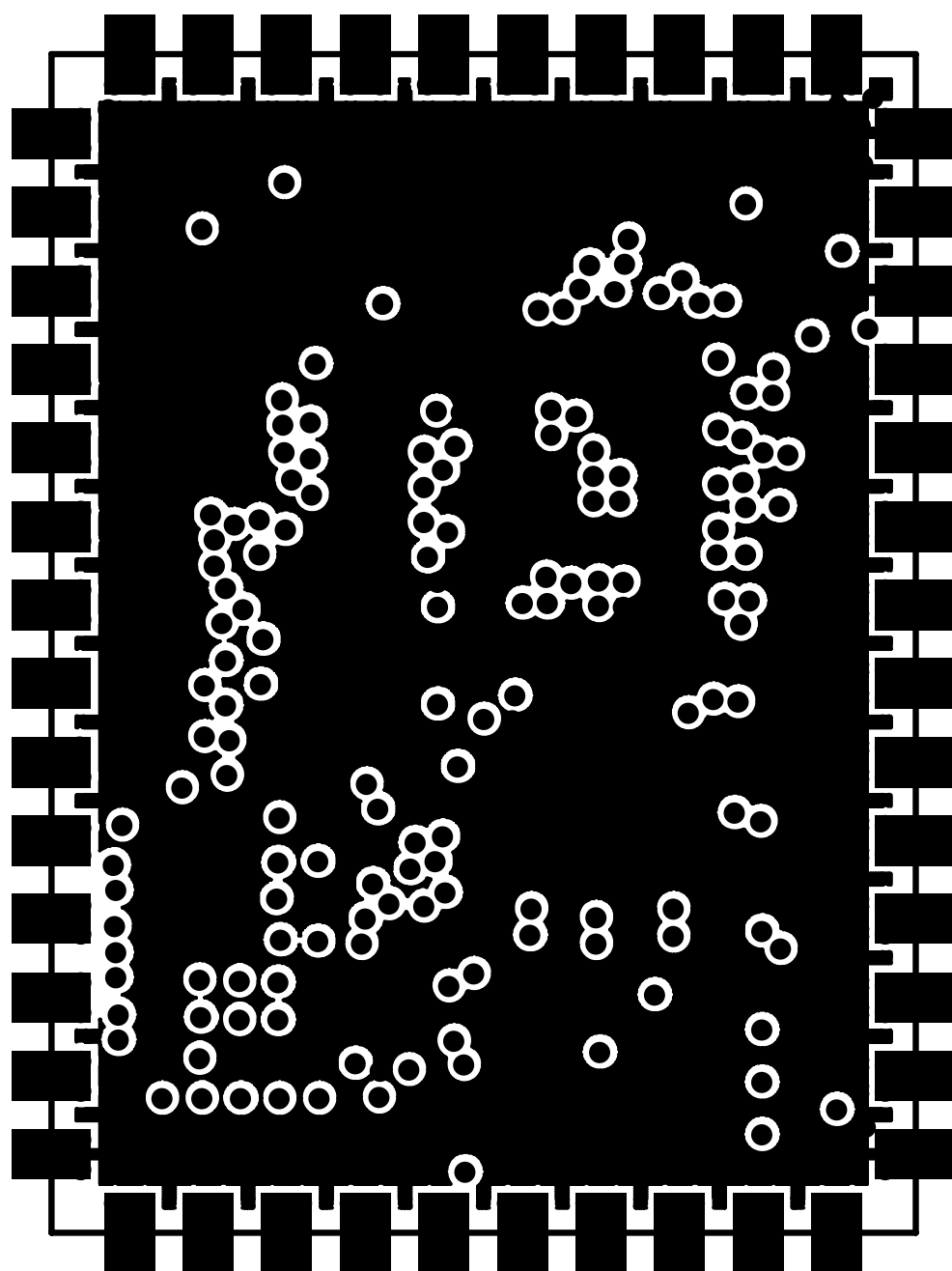
Mid Layer 1
