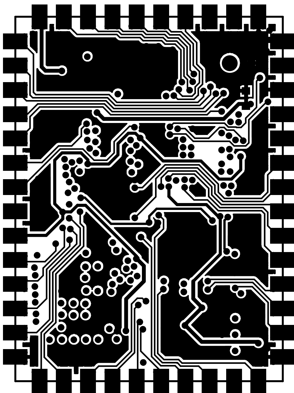
Bottom Layer
