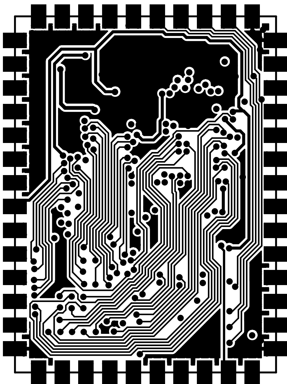
Mid Layer 2
