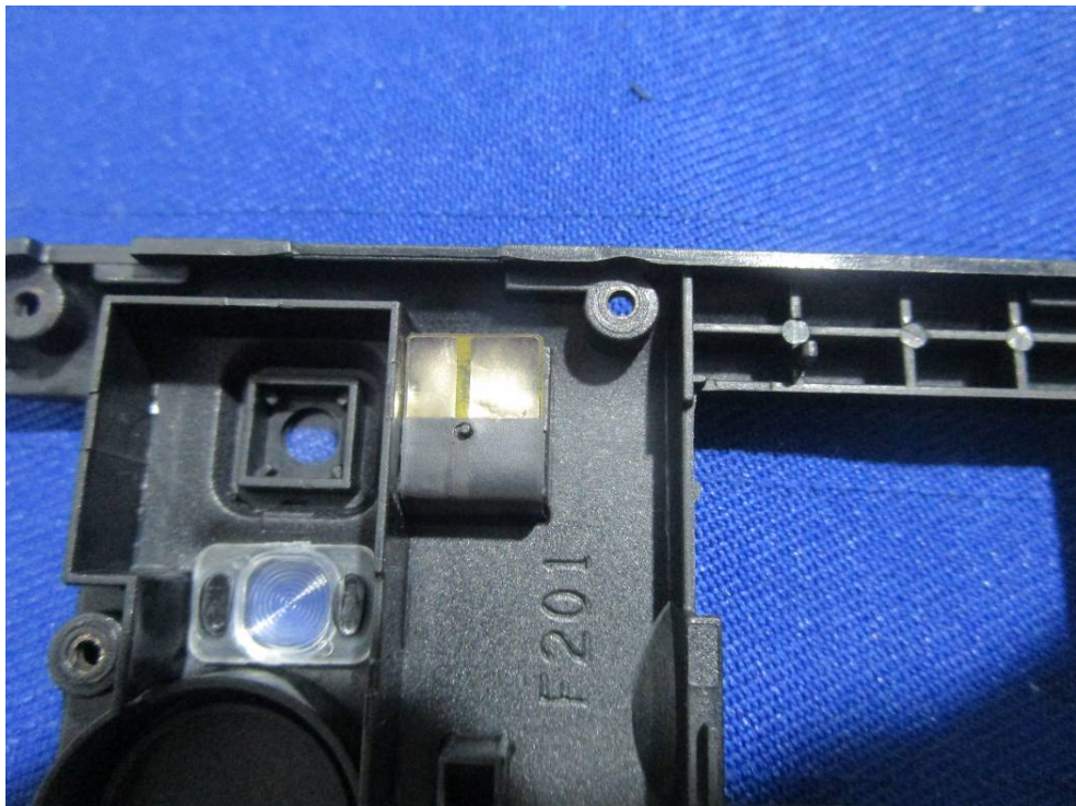
GSM Antenna
