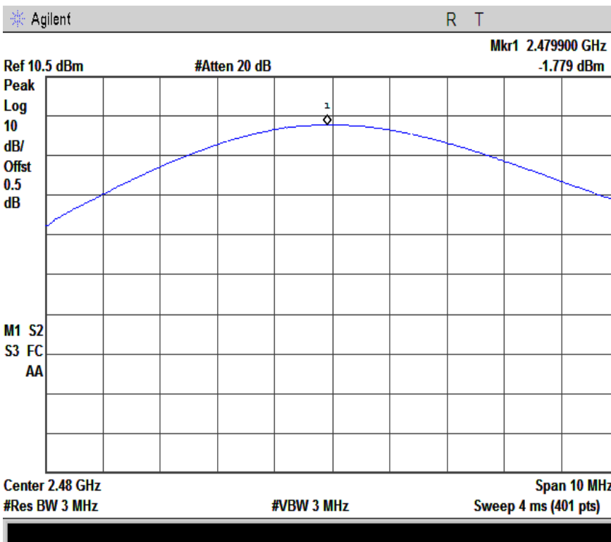
3M-power-2480
