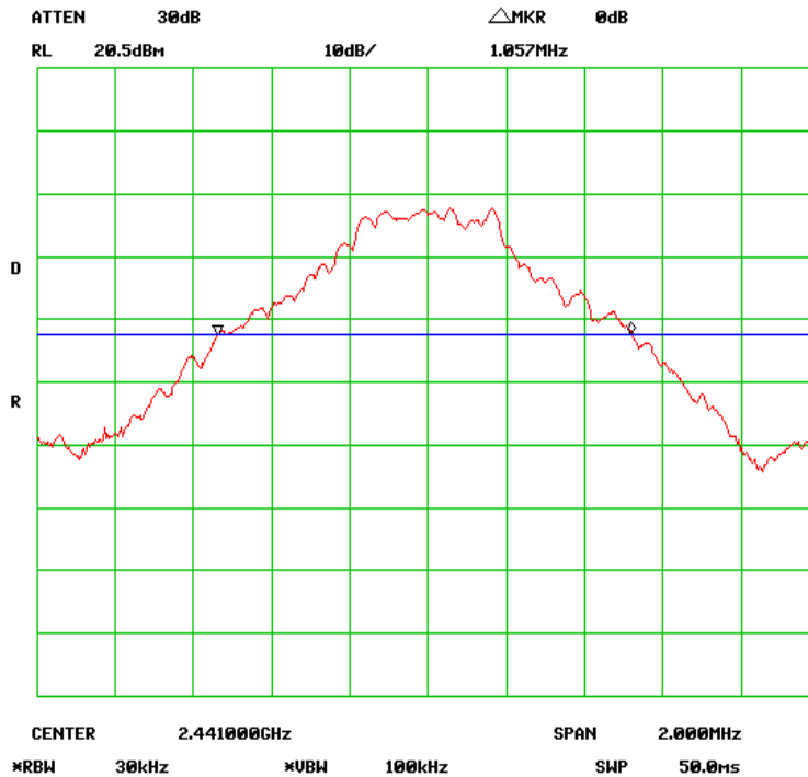
1M-20dB-2441
