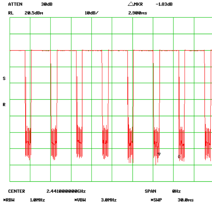
DH5-2441
