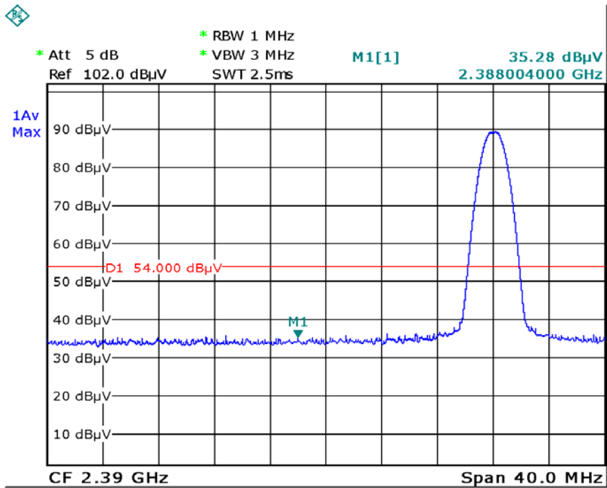
1M-Left Side-AV
