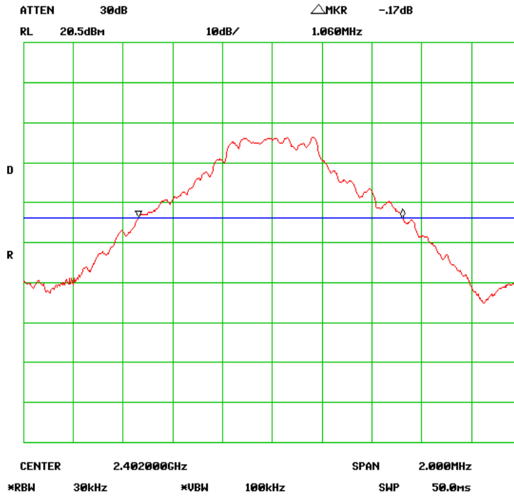
1M-20dB-2402
