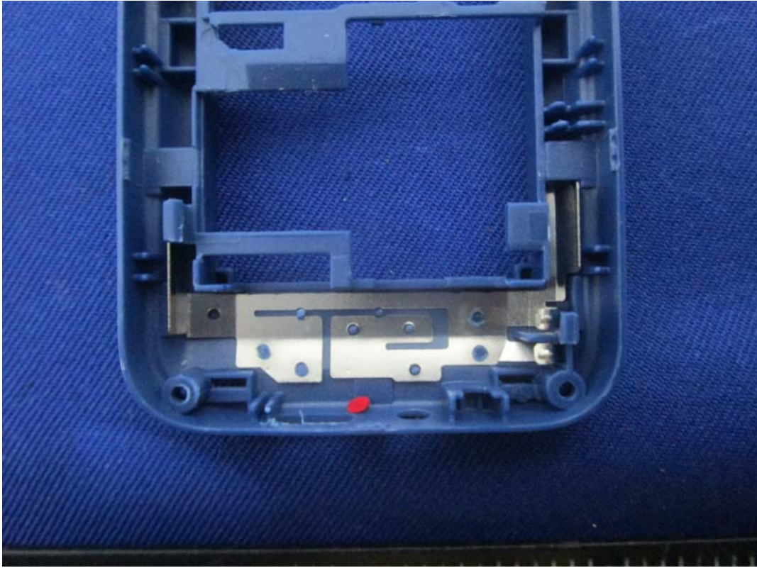
GSM Antenna
