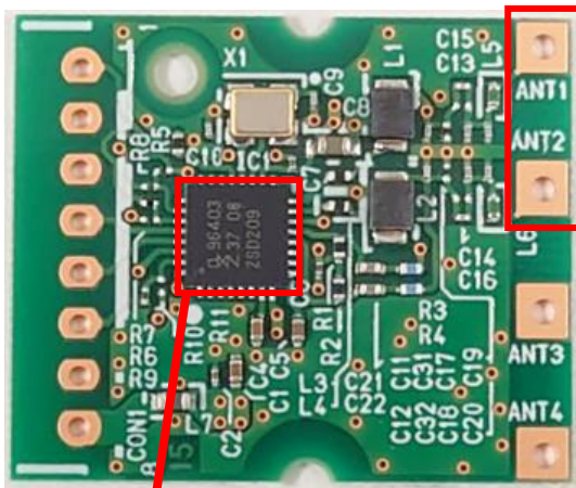
RF IC
