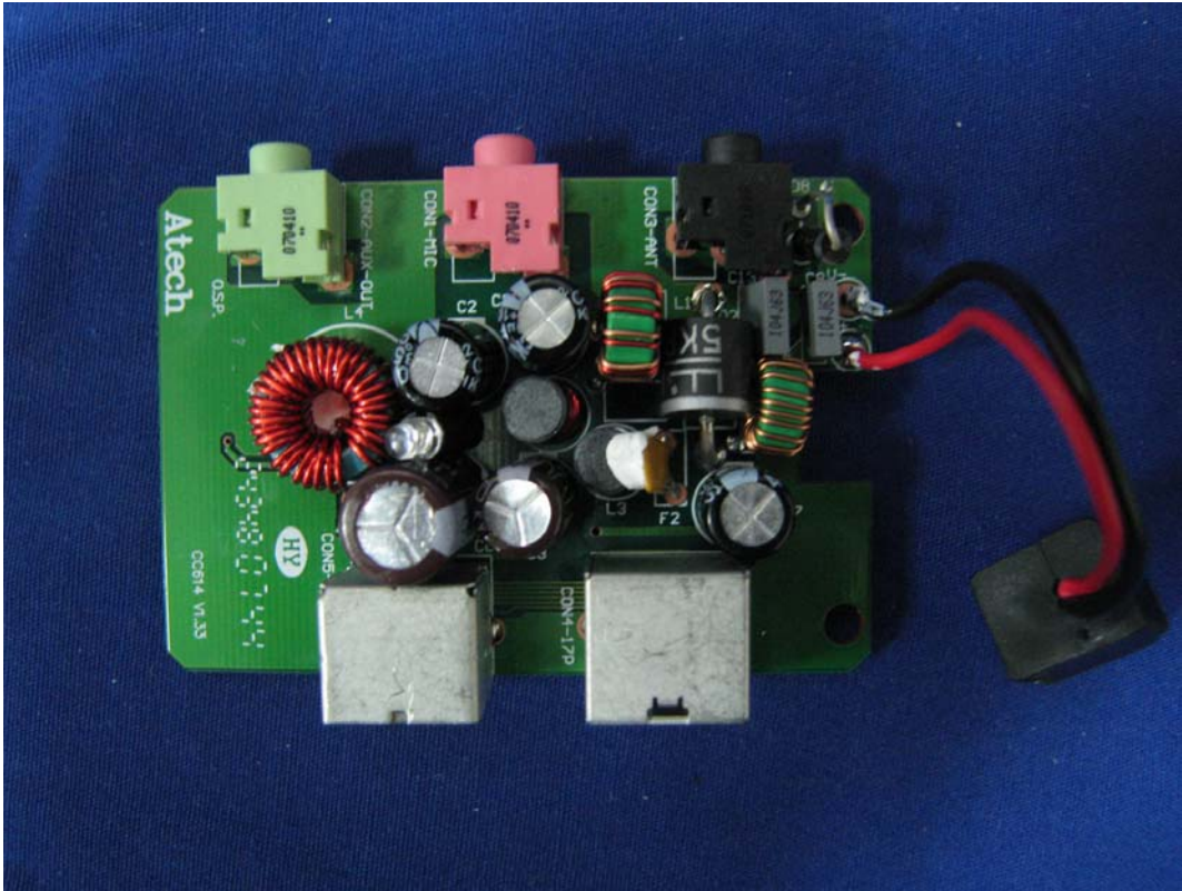
(53) EUT Photo
