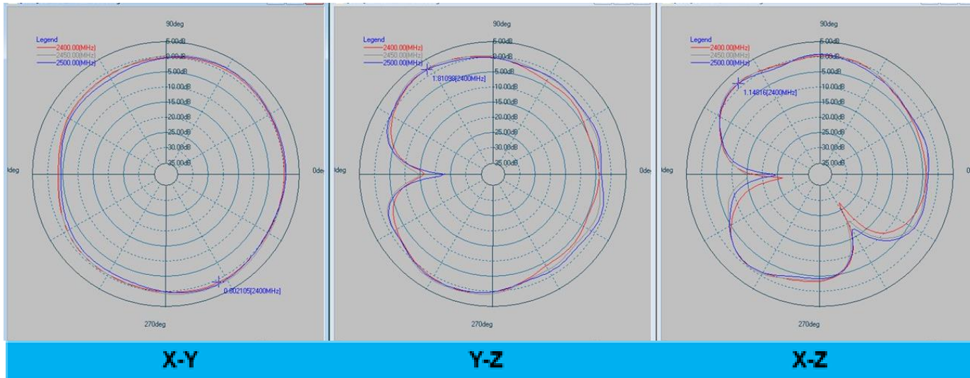
WN4649L module
