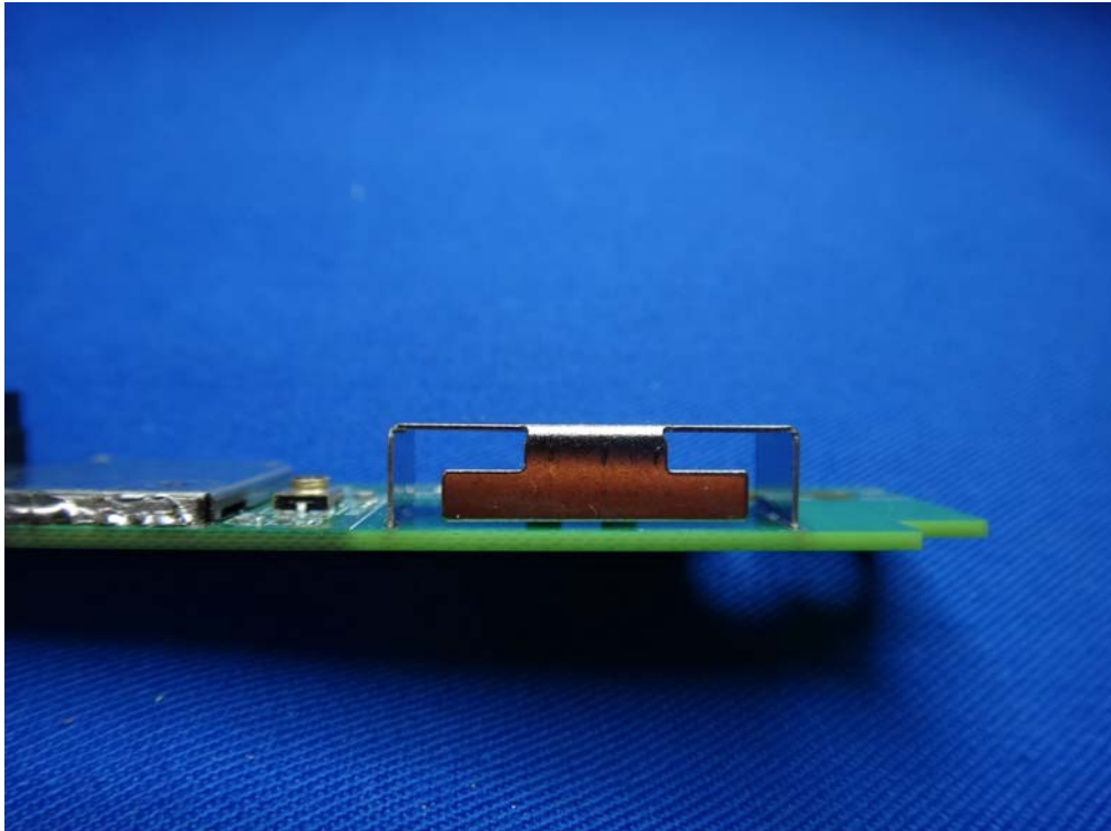
(5) EUT Photo (Antenna: Auden)
