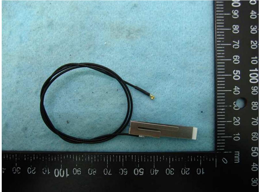
Ant. 4: 500mm
