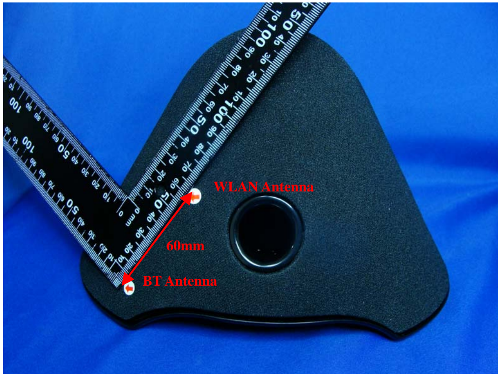
(49) EUT Photo
