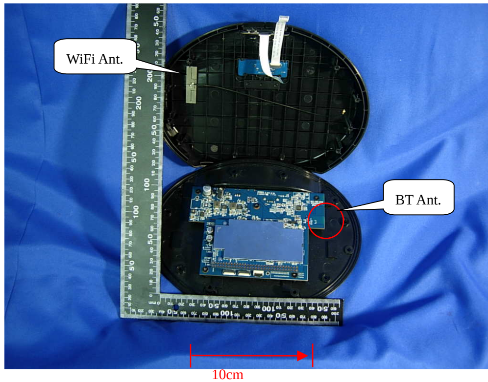
(5) EUT Photo
