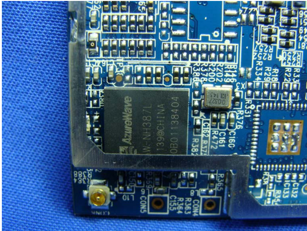
(37) EUT Photo
