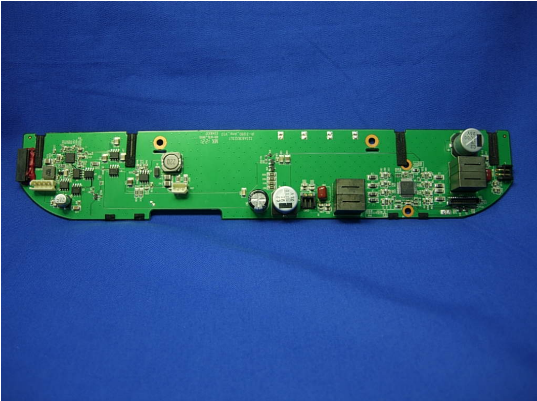
(37) EUT Photo
