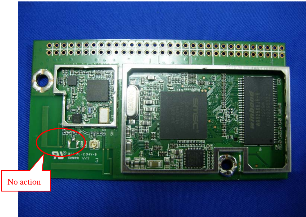
(4) EUT Photo
