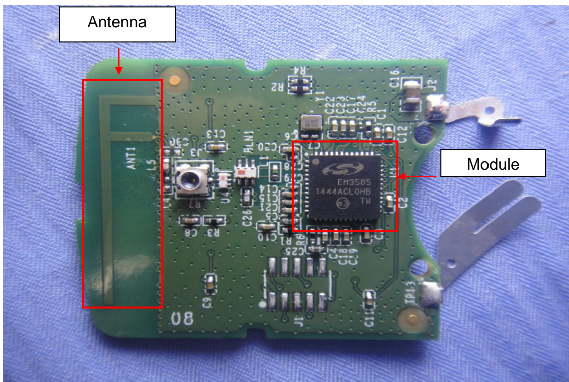
Antenna & Module
