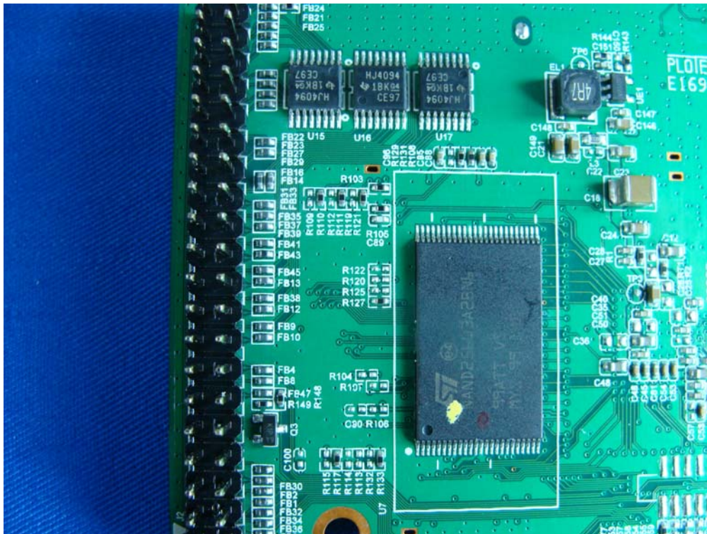
(21) EUT Photo
