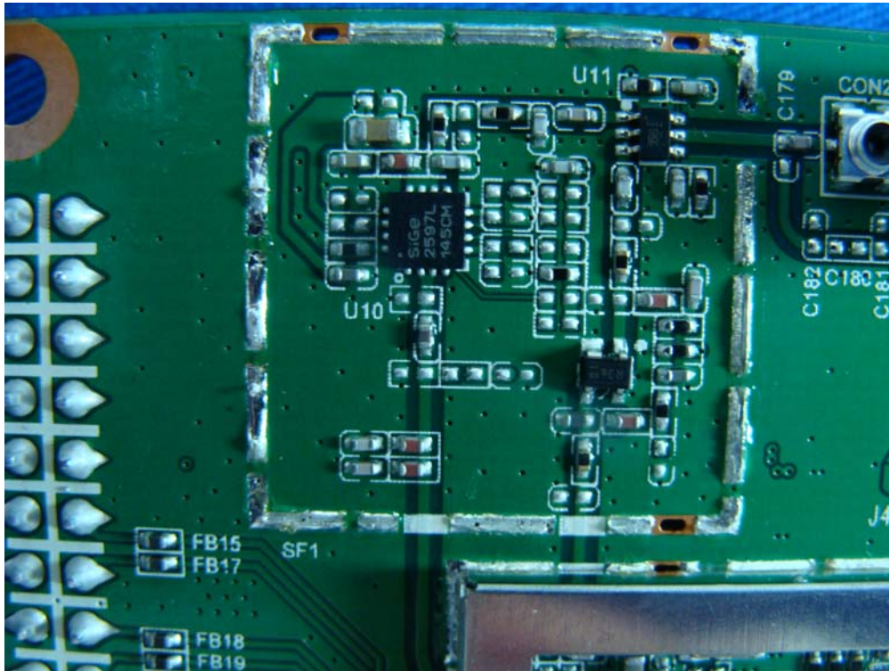
(17) EUT Photo
