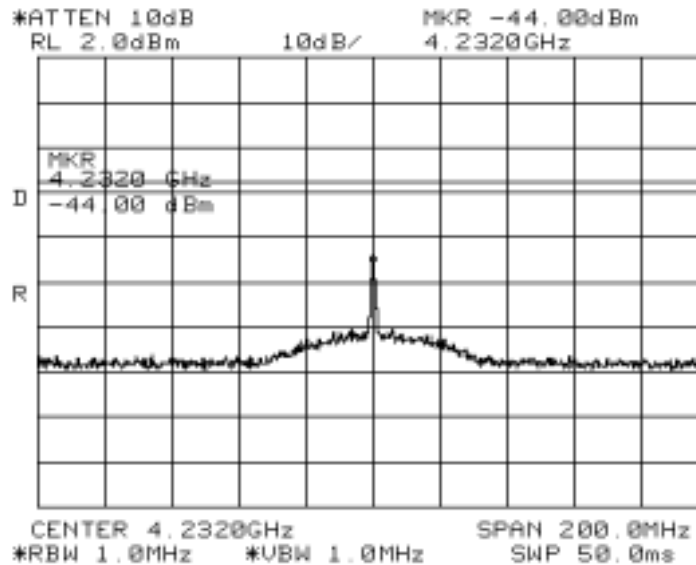
T45029 / 1022 (4 GHz)
