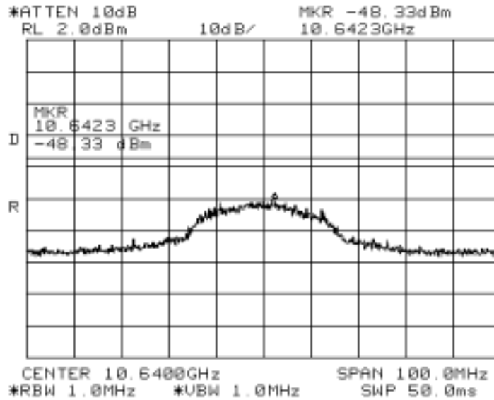
T45029 / 814
