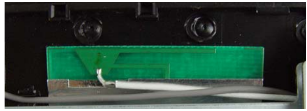
Tx2 Antenna
