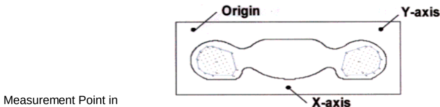
Fig. 13. SAR Area Scan
