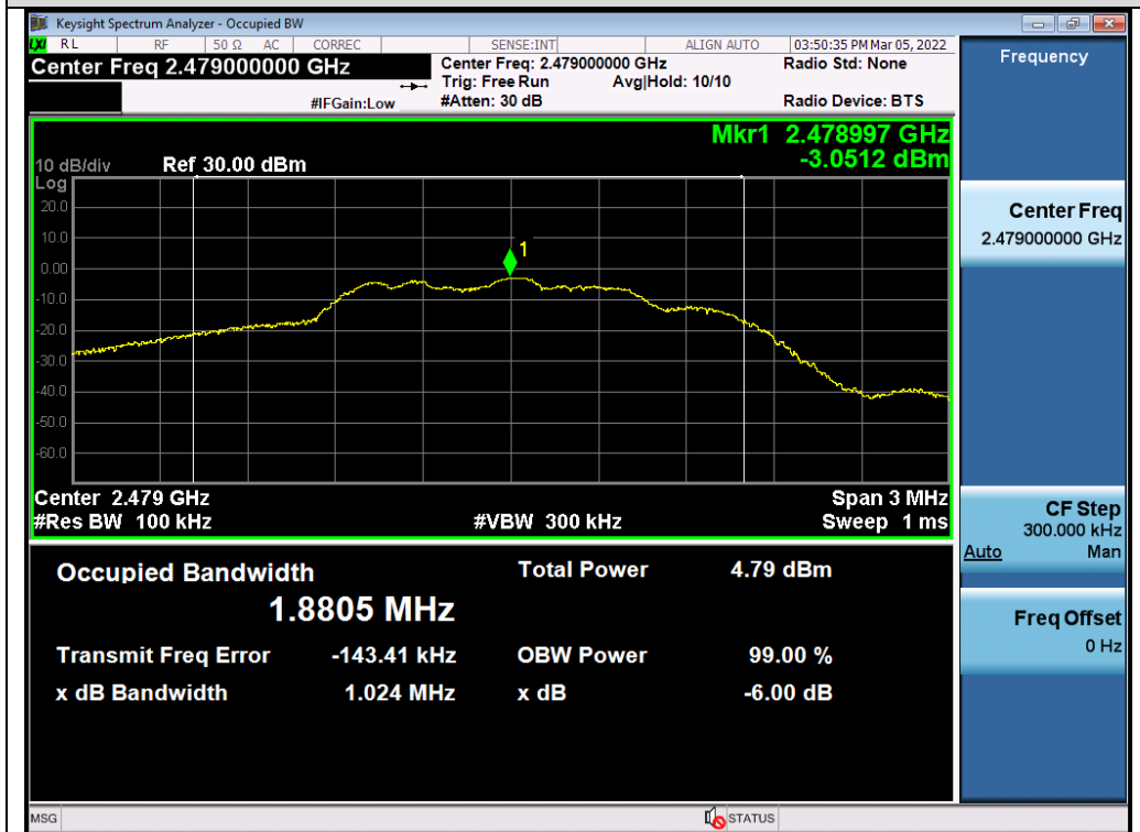
Test_Graph_2.4GHz_ANT1_2479_GFSK_DTSSBW
