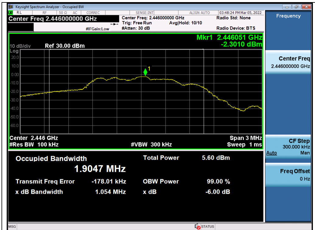
Test_Graph_2.4GHz_ANT1_2446_GFSK_DTSSBW
