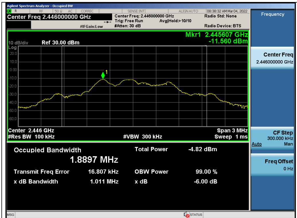
Test_Graph_GFSK_ANT1_2446_DTSBW
