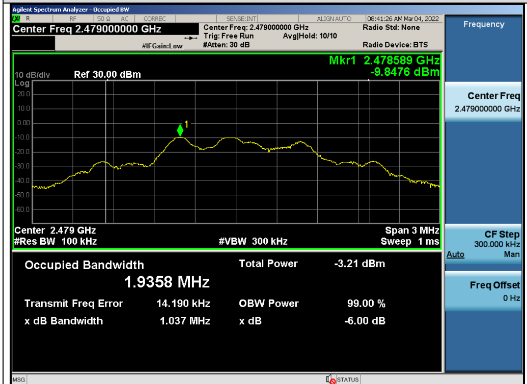
Test_Graph_GFSK_ANT1_2479_DTSBW
