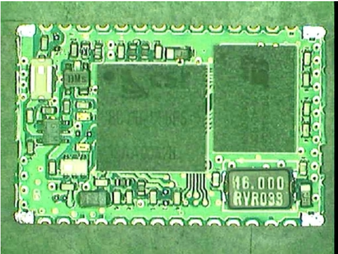
PCB top
