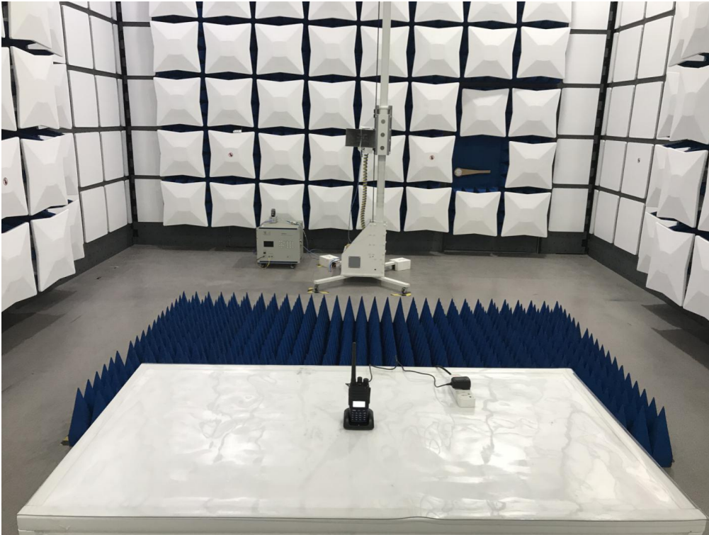
Antenna 2:Rx: 220MHz-260MHz
