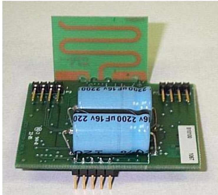
Antenna: Rear
