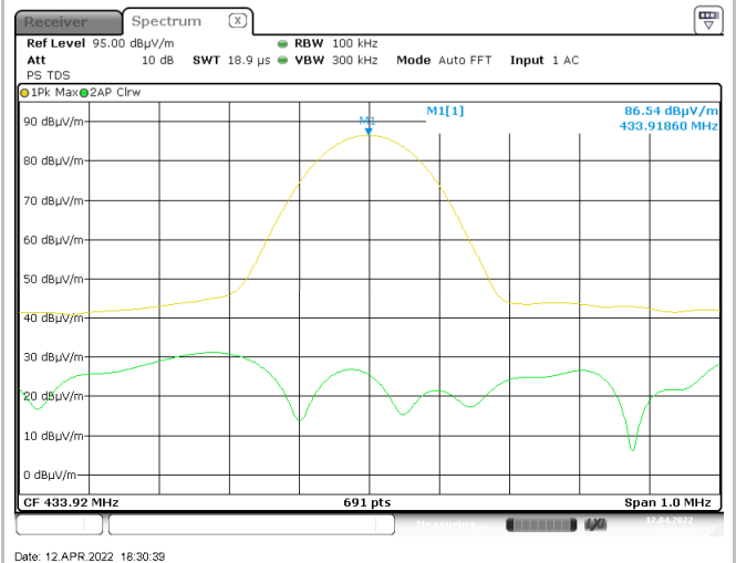
Plot 2 – OOK modulation
