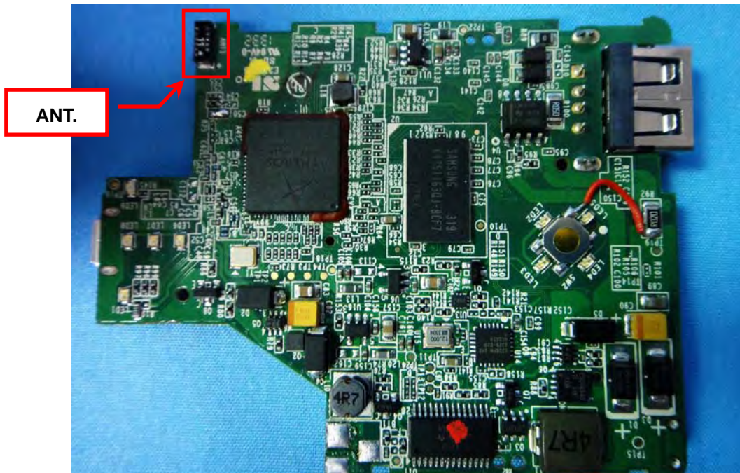
EUT Photo 4 )
