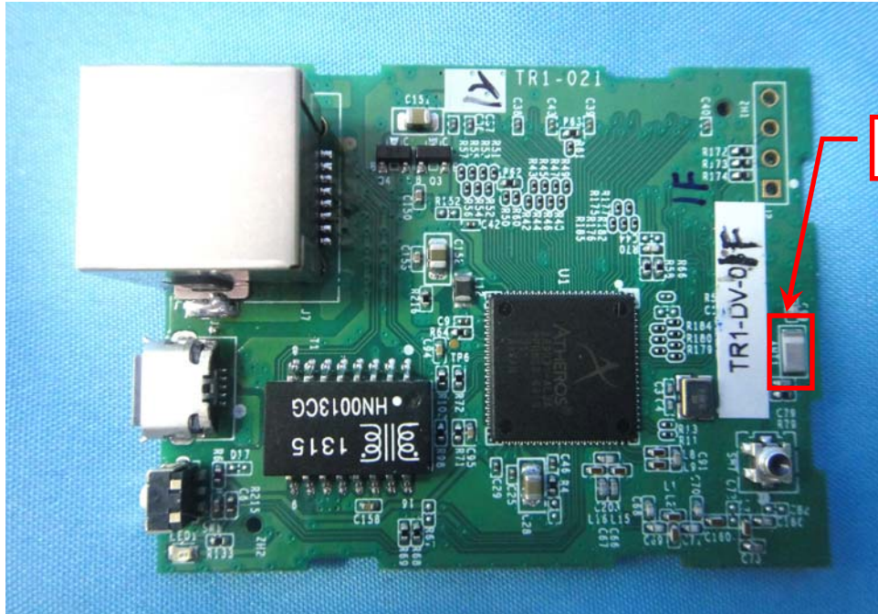
EUT Photo 3 )
