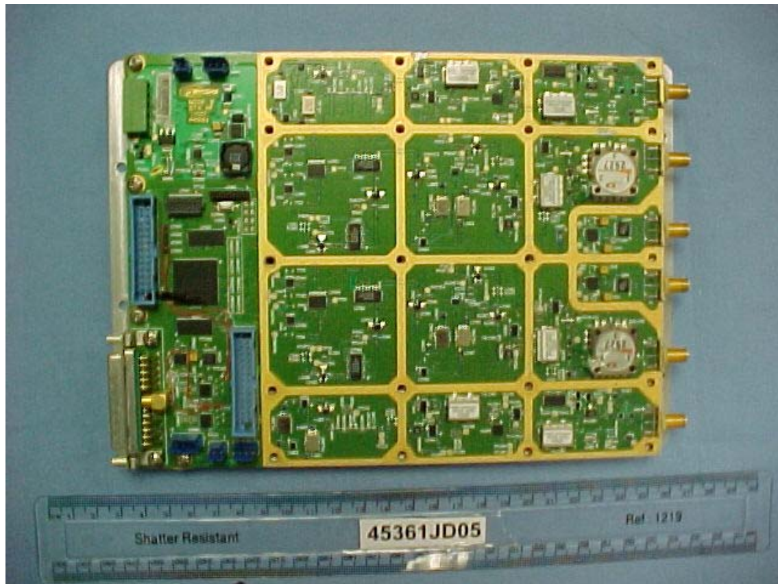
DZ PCB1 Side 1
