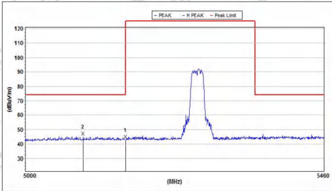
5260MHz Horizontal
