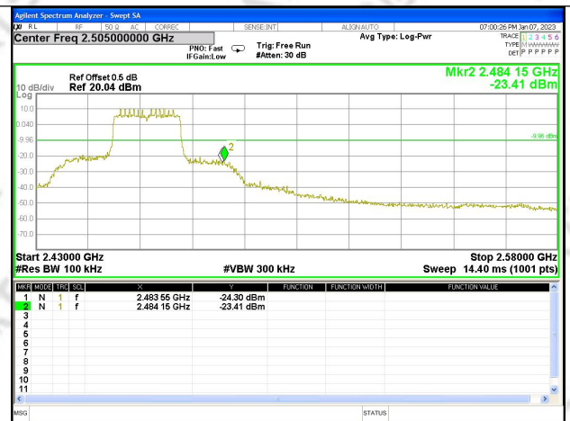
CH11_Ant. 1
