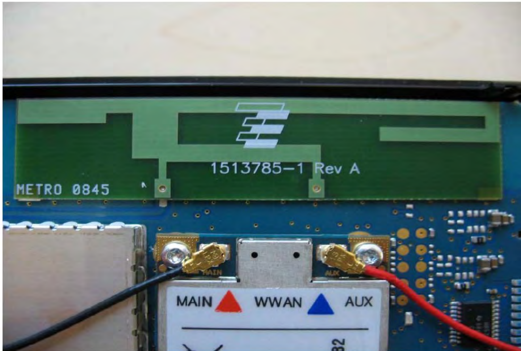
UMTS module
