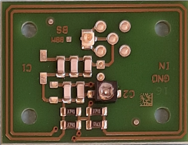
Top side
