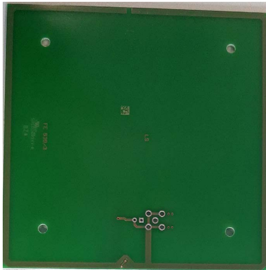
Bottom Side
