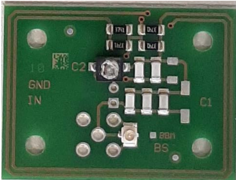
Top Side
