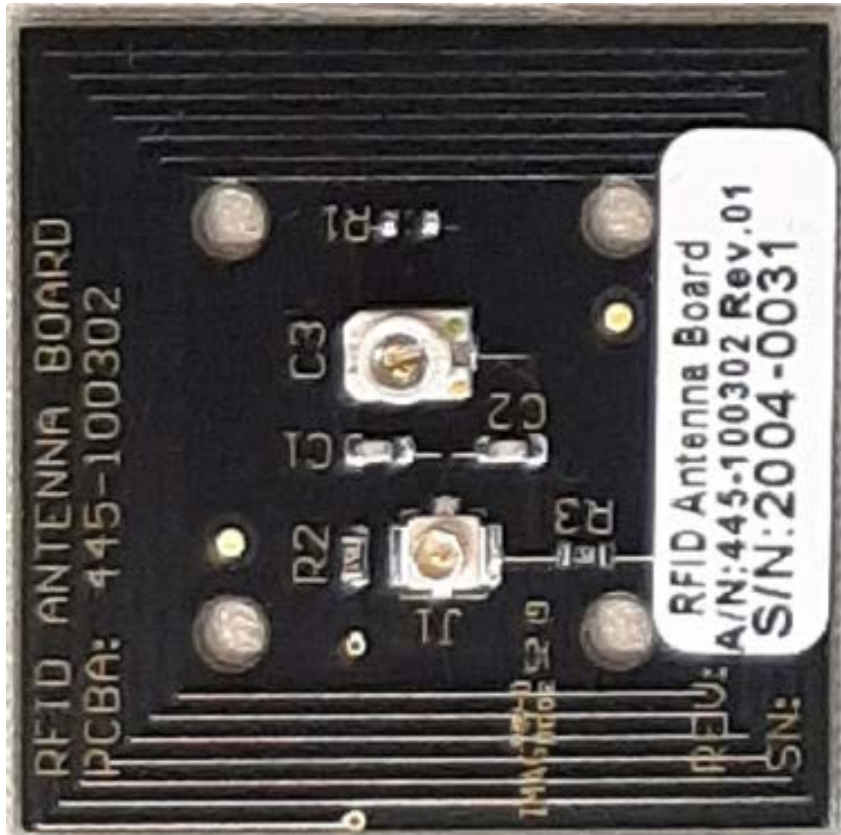
Top Side
