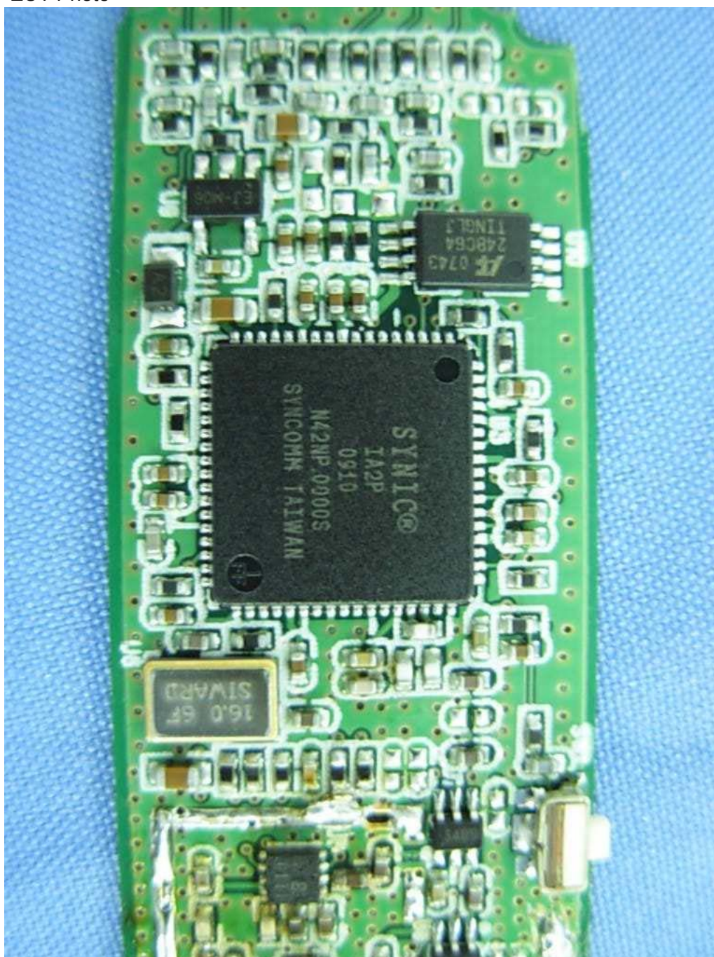
(10) EUT Photo
