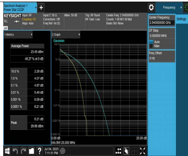
Band41-10MHz-QPSK-40640-50RB#0
