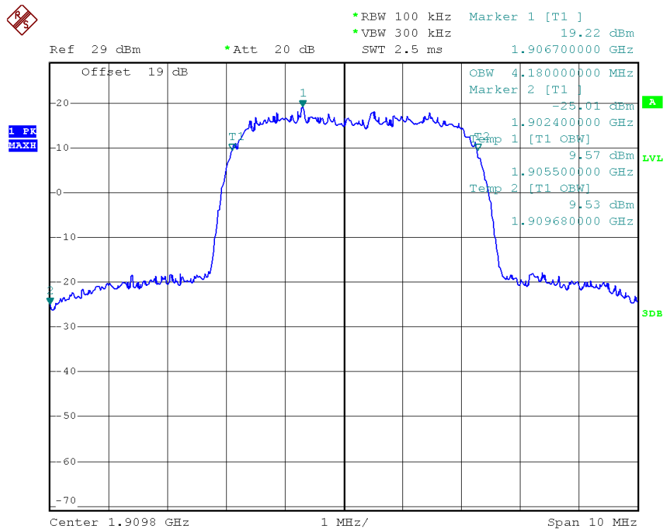
(Plot F: WCDMA1900MHz Channel = 9538)
