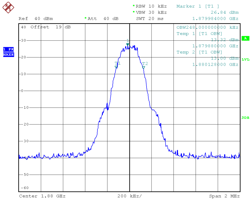
(Plot W: GPRS 1900MHz Channel = 661)
