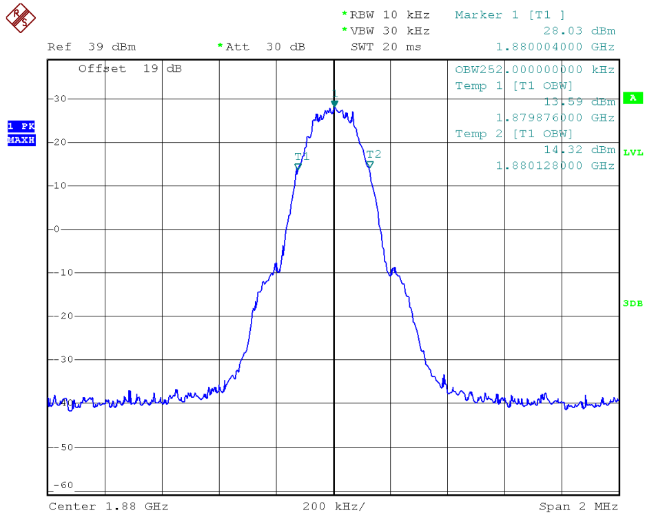
(Plot Q: GSM 1900MHz Channel = 661)
