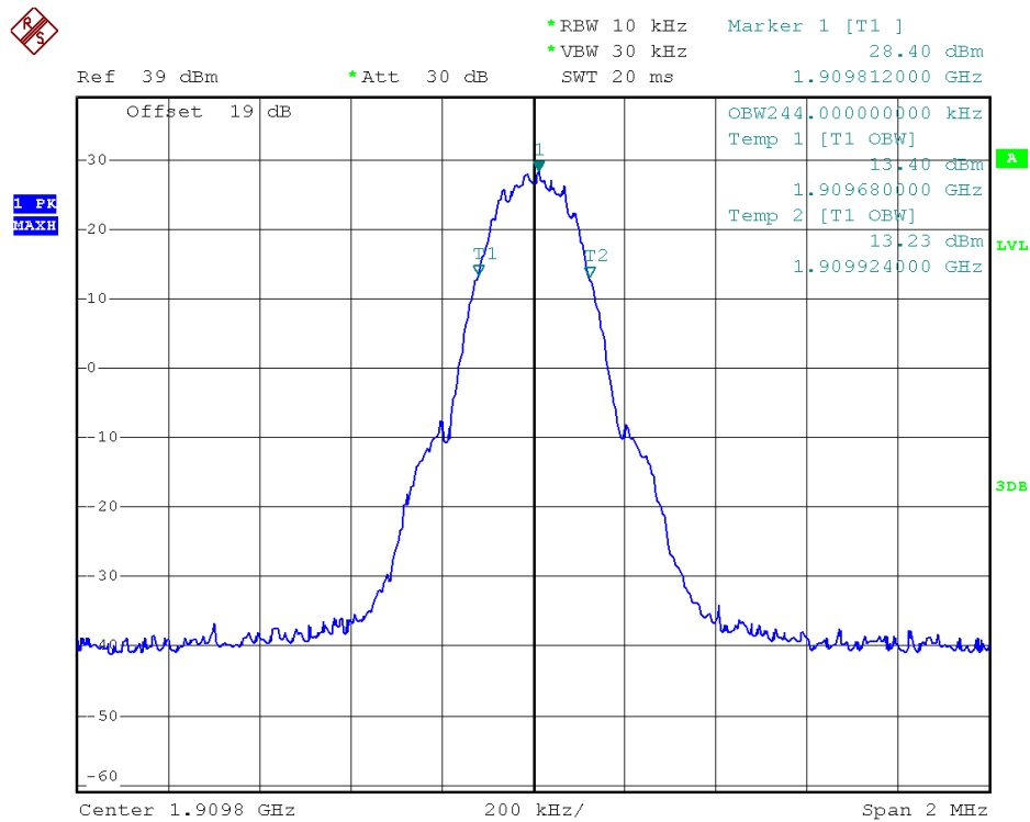
(Plot D1: EDGE 1900MHz Channel = 810)
