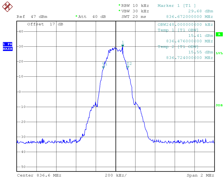
(Plot N: GSM 850MHz Channel = 190)
