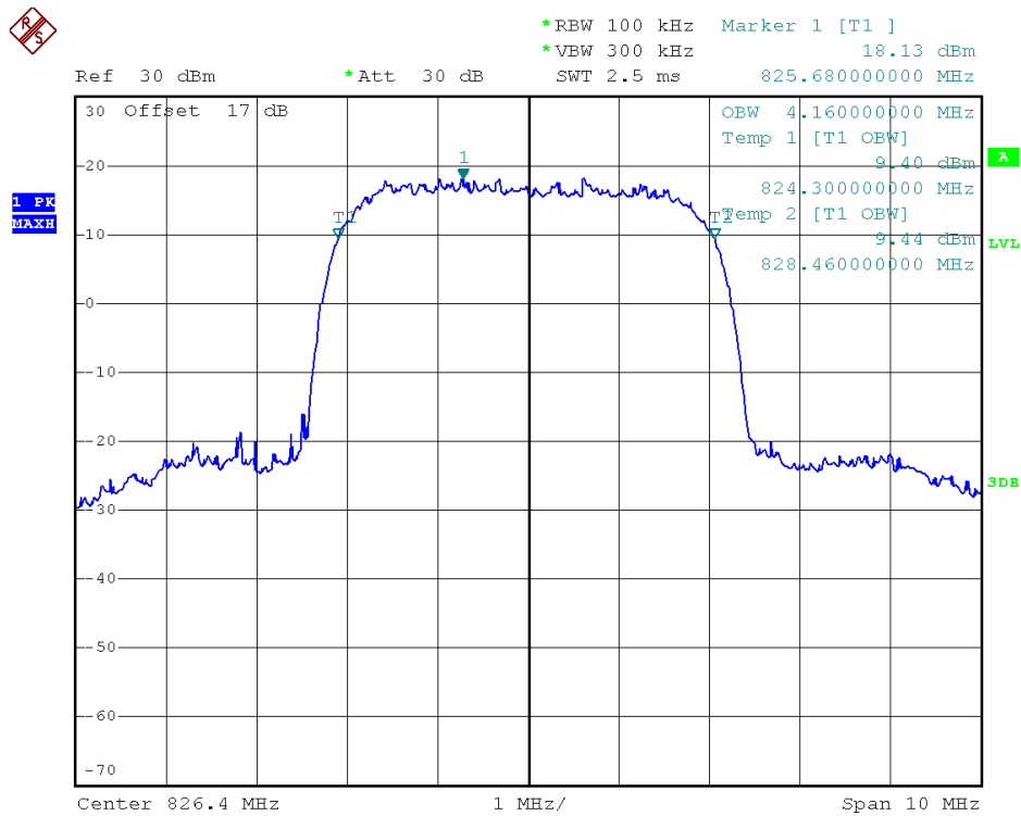
(Plot A: WCDMA 850MHz Channel = 4132)
