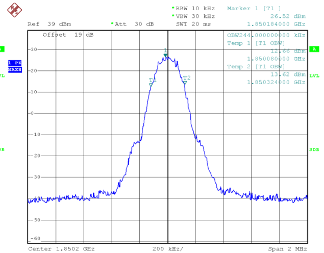
(Plot J: GPRS 1900MHz Channel = 512)
