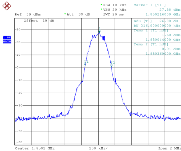
(Plot J: GPRS 1900MHz Channel = 512)
