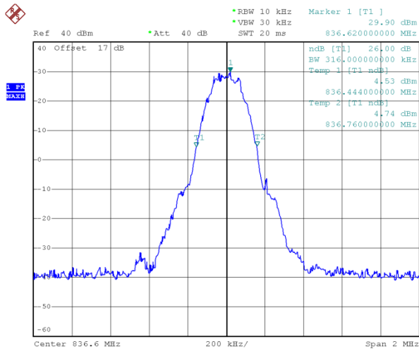
(Plot B: GSM 850MHz Channel = 190)
